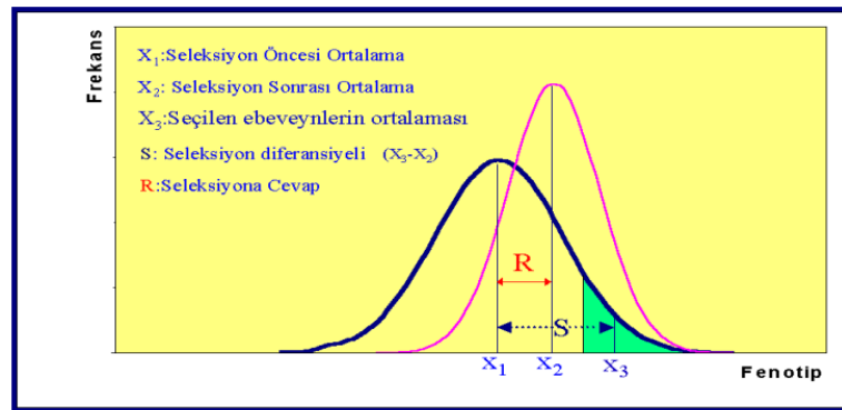
Şekil 1. Seleksiyon öncesi ve sonrası popülasyon varyansındaki ve ortalamasındaki değişim (Öztürk, 2000).
